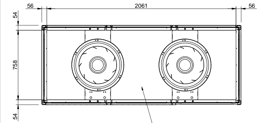
SEZIONE A-A
